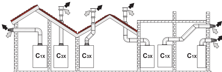
wygląd 31- Przykłady połączenia przewodami współosiowymi (⇨ = Powietrze / ⇨ = Spaliny)
