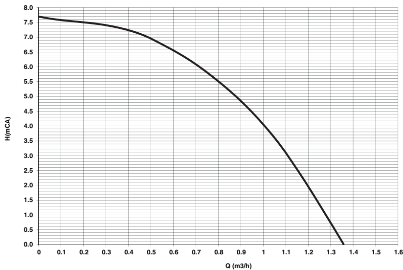
εικ. 66- Διαθέσιμο υπολειπόμενο μανομετρικό ύψος στην εγκατάσταση
