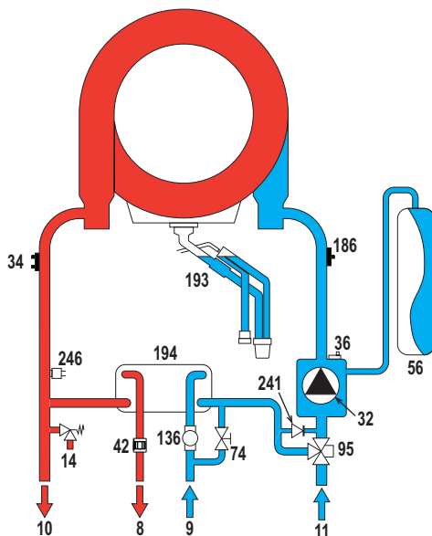
wygląd 64- Obieg wody
