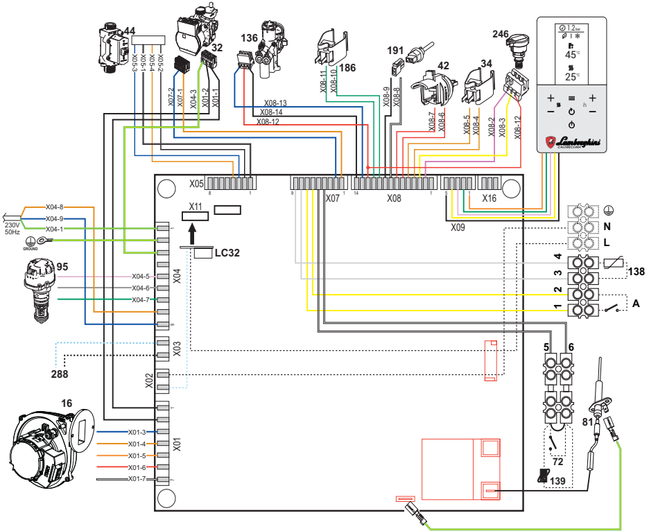
fig. 66- Schema electrică
