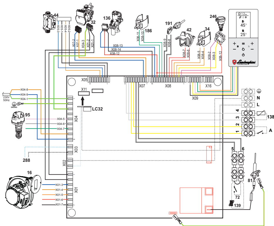
fig. 66- Esquema eléctrico
