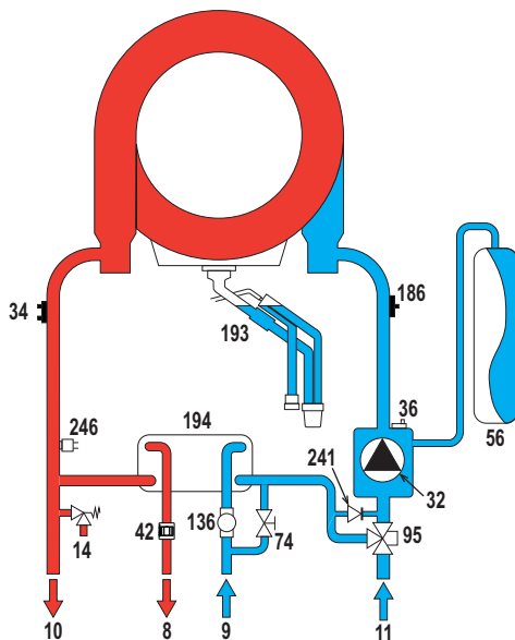
fig. 64 - Circuito idraulico
