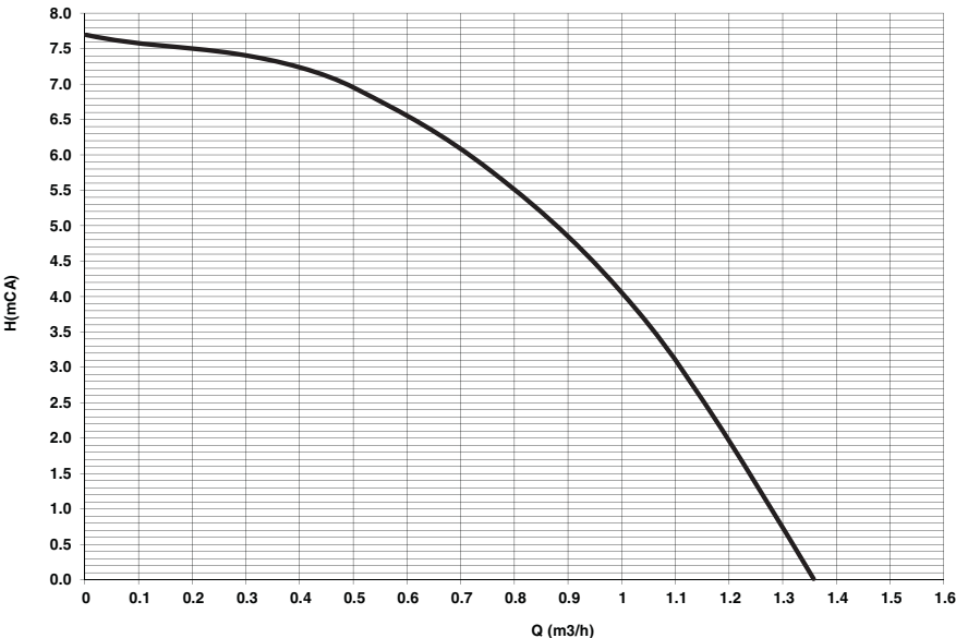
fig. 65- Carga hidrostática residual disponible en la instalación
