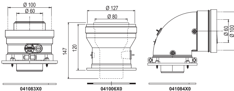
wygląd 32- Akcesoria wyjściowe do przewodów współosiowych
