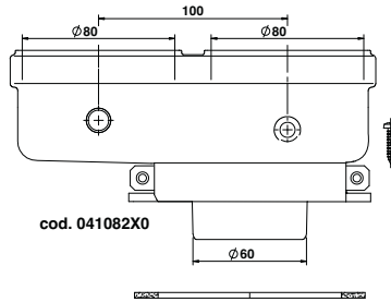
fig. 34- Accesorio inicial para conductos separados
