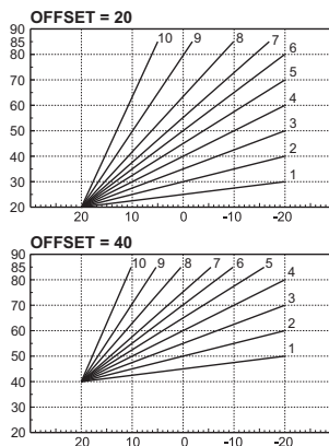
wygląd 25- Przykład równoległego przesunięcia krzywych kompensacji
