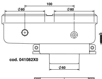
εικ. 34- Εξάρτημα σύνδεσης για ξεχωριστούς αγωγούς
