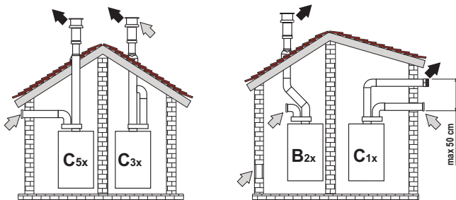
fig. 33- Exemple de racordare cu tuburi separate (□ = Aer / ■ = Gaze arse)
