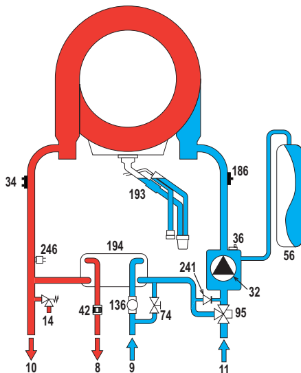
εικ. 64- Υδραυλικό κύκλωμα
