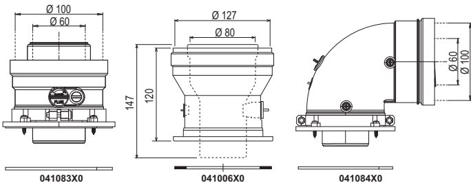
fig. 32- Accesorios iniciales para conductos coaxiales
