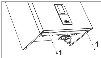
fig. 42 - Apertura pannello frontale
