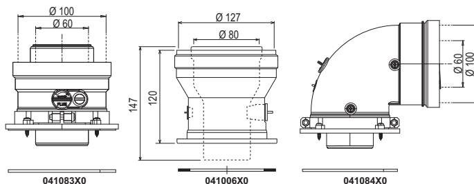
fig. 32 - Accessori di partenza per condotti coassiali
