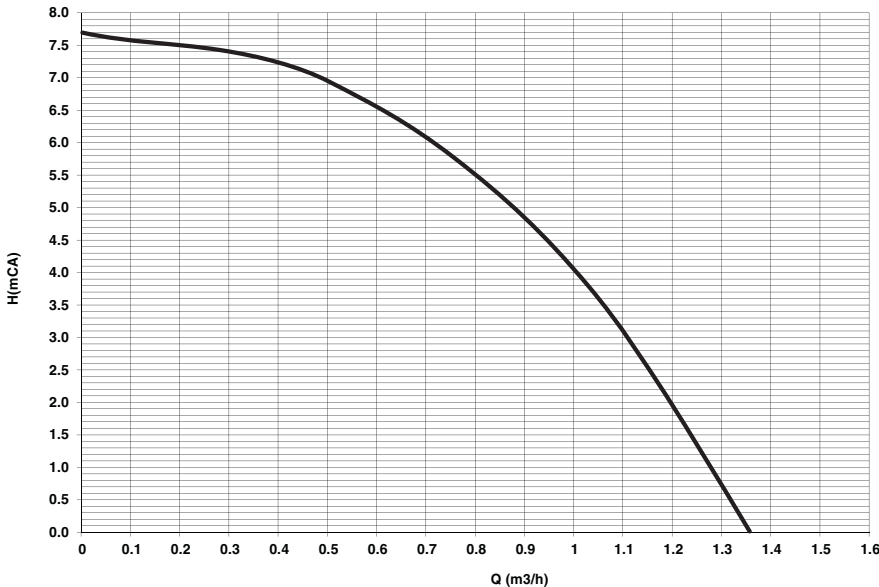
fig. 65 - Prevalenza residua disponibile all'impianto
