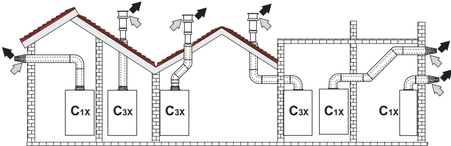
fig. 31- Ejemplos de conexión con tubos coaxiales (⇨ = aire / ⇨ = humos)
