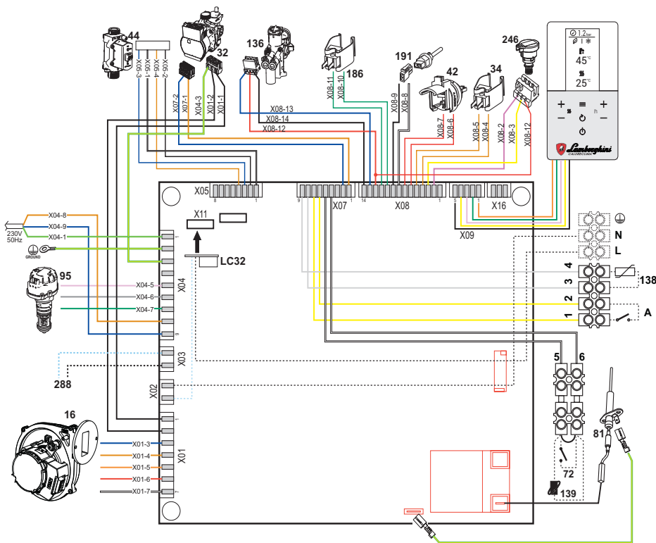
fig. 67 - Schema elettrico
